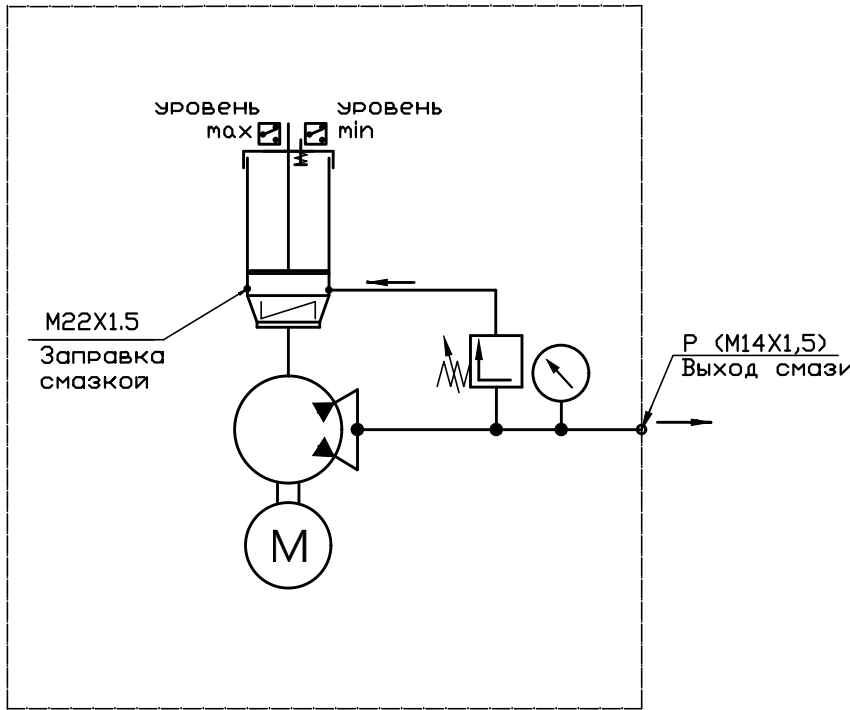
Схема гидравлическая
