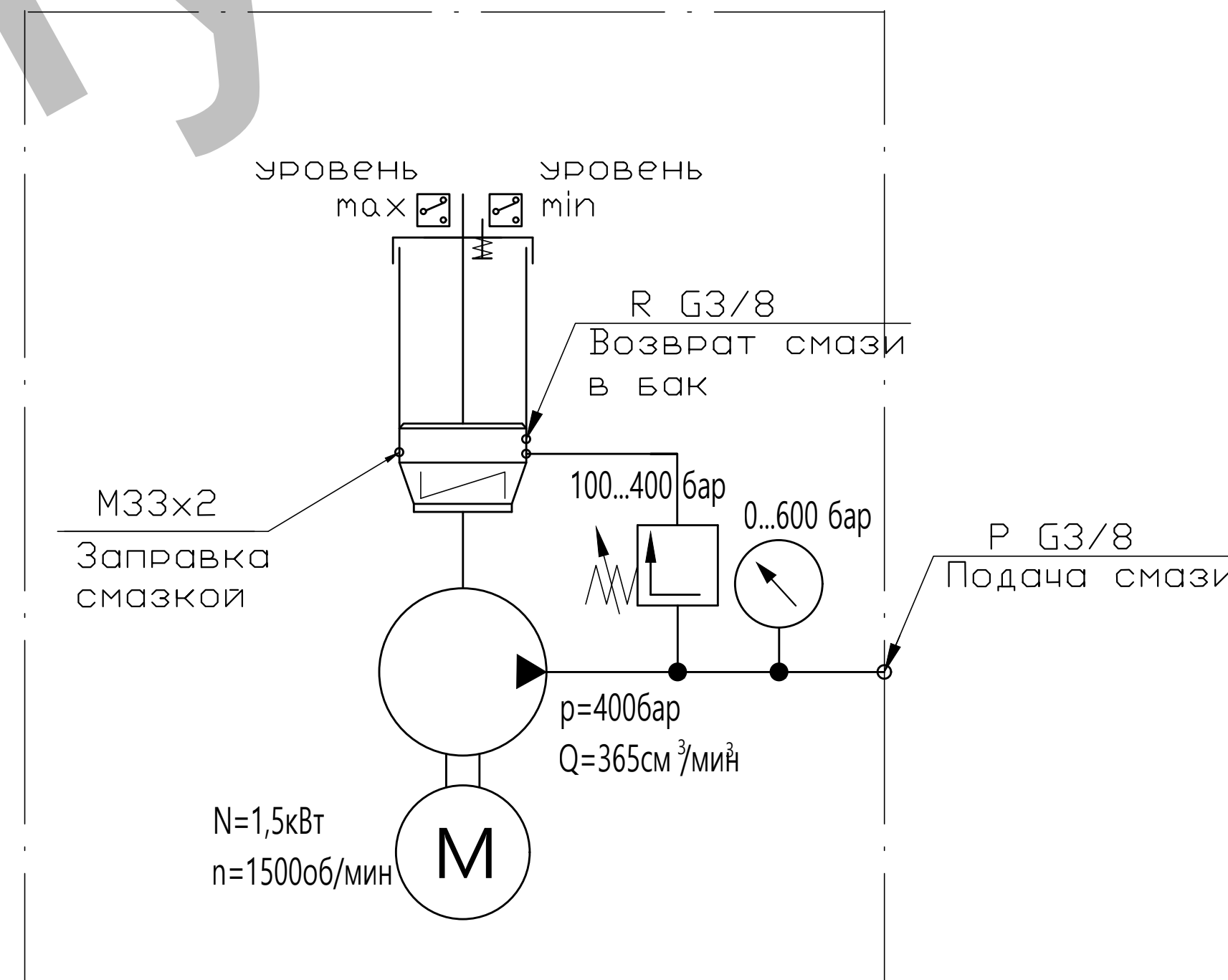
Схема гидравлическая
