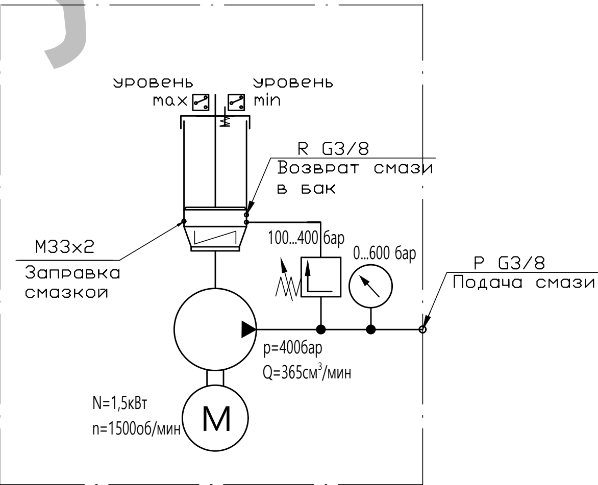
Схема гидравлическая
