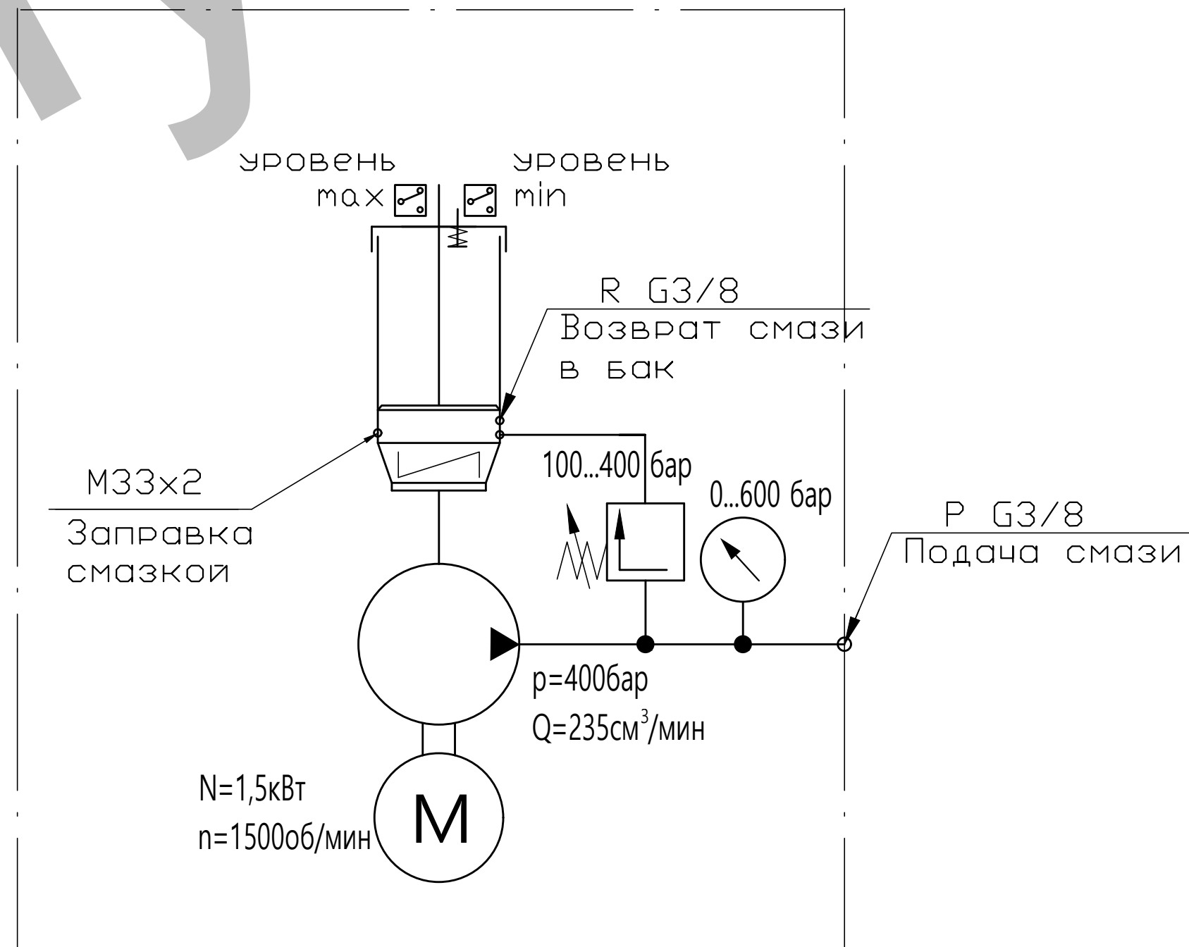
Схема гидравлическая
