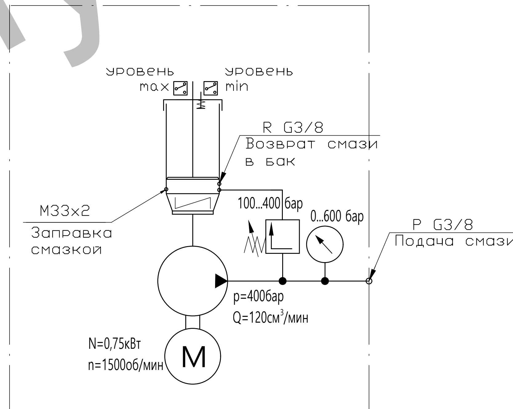
Схема гидравлическая
